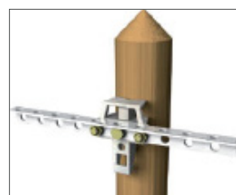
Installation de traverse
